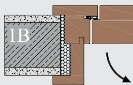
Блок-рама с полукоробкой, монтаж на стену. Открывание внутрь.
