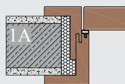
Разъемная коробка с монтажом на стену. Ширина наличника 63/75 мм.
